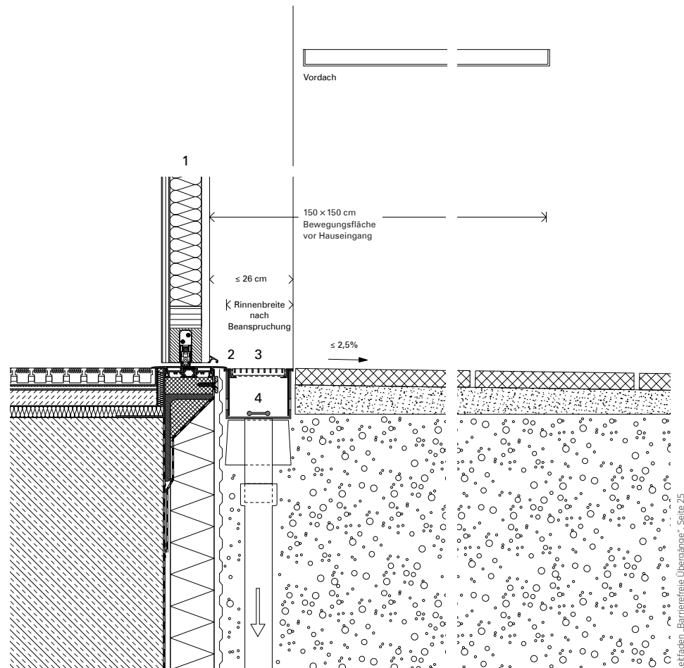
Detail schwellenfreier Zugang Haustür
